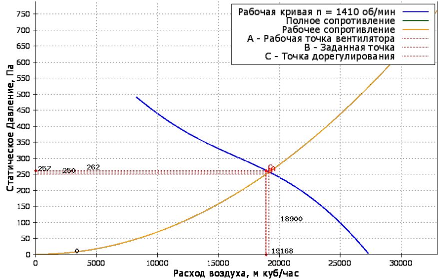
Вентилятор осевой крышный VOP 80-4х15
