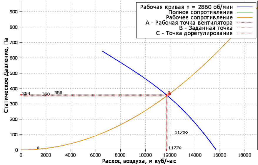
Вентилятор осевой крышный VOP 56-3х30
